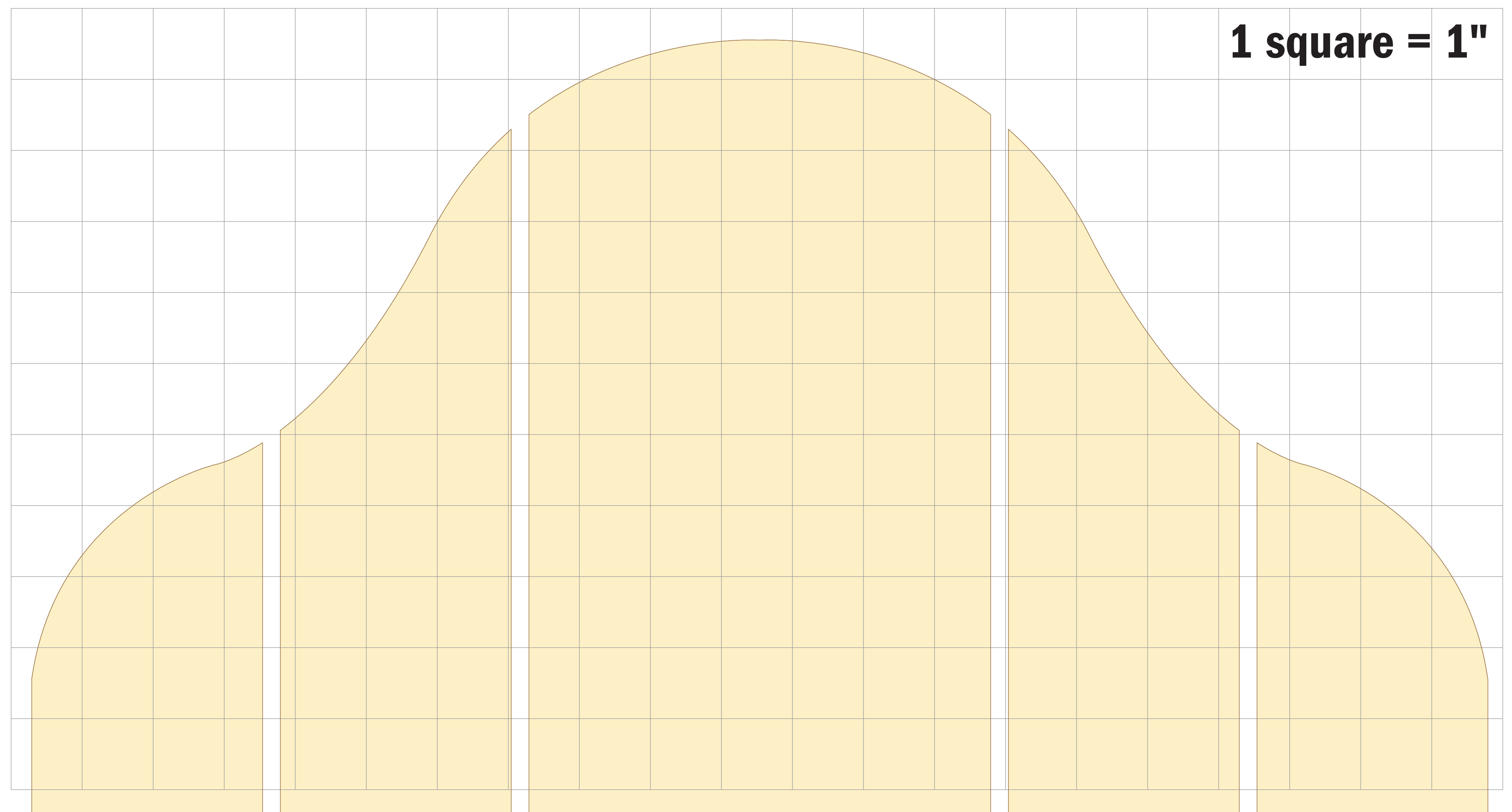
BACKREST SLATS
